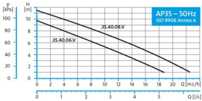
Charakterystyka Grundfos Unilift AP35
