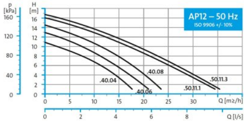
Charakterystyka Grundfos Unilift AP12
