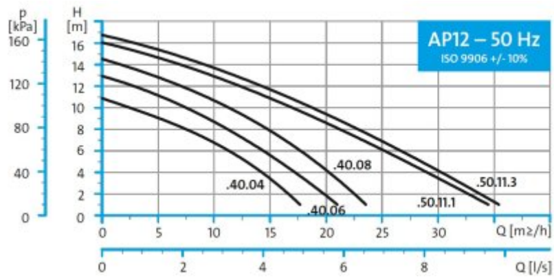
Charakterystyka Grundfos Unilift AP12
