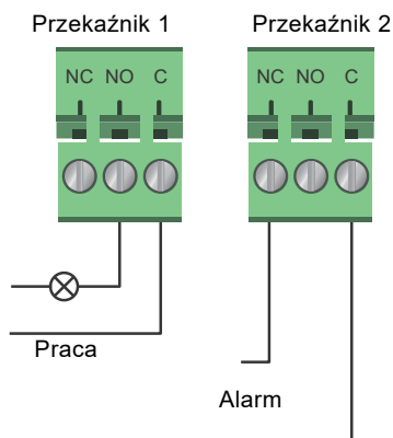
Rys. 46 Wyjście przełącznikowe
