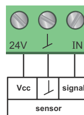
Rys. 49 Wejście analogowe dla przetwornika zewn., 0-10 V
