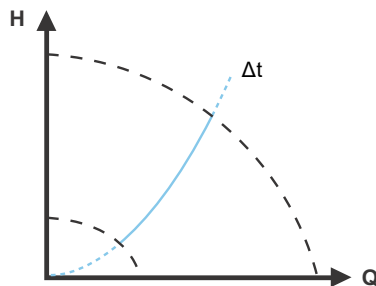
Rys. 33 Różnica temperatur
