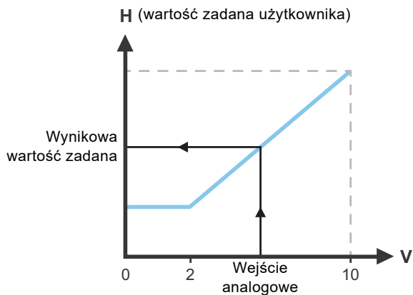
Rys. 54 "Liniowa z MIN", 0-10 V
