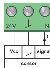
Rys. 50 Wejście analogowe dla przetwornika zewn., 4-20 mA
