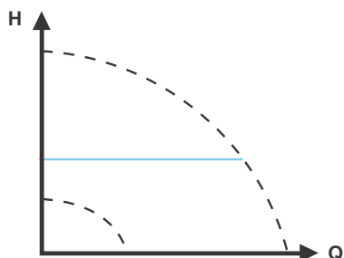
Rys. 29 Stałe ciśnienie
