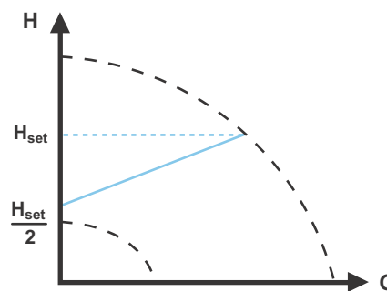
Rys. 28 Ciśnienie proporcjonalne
