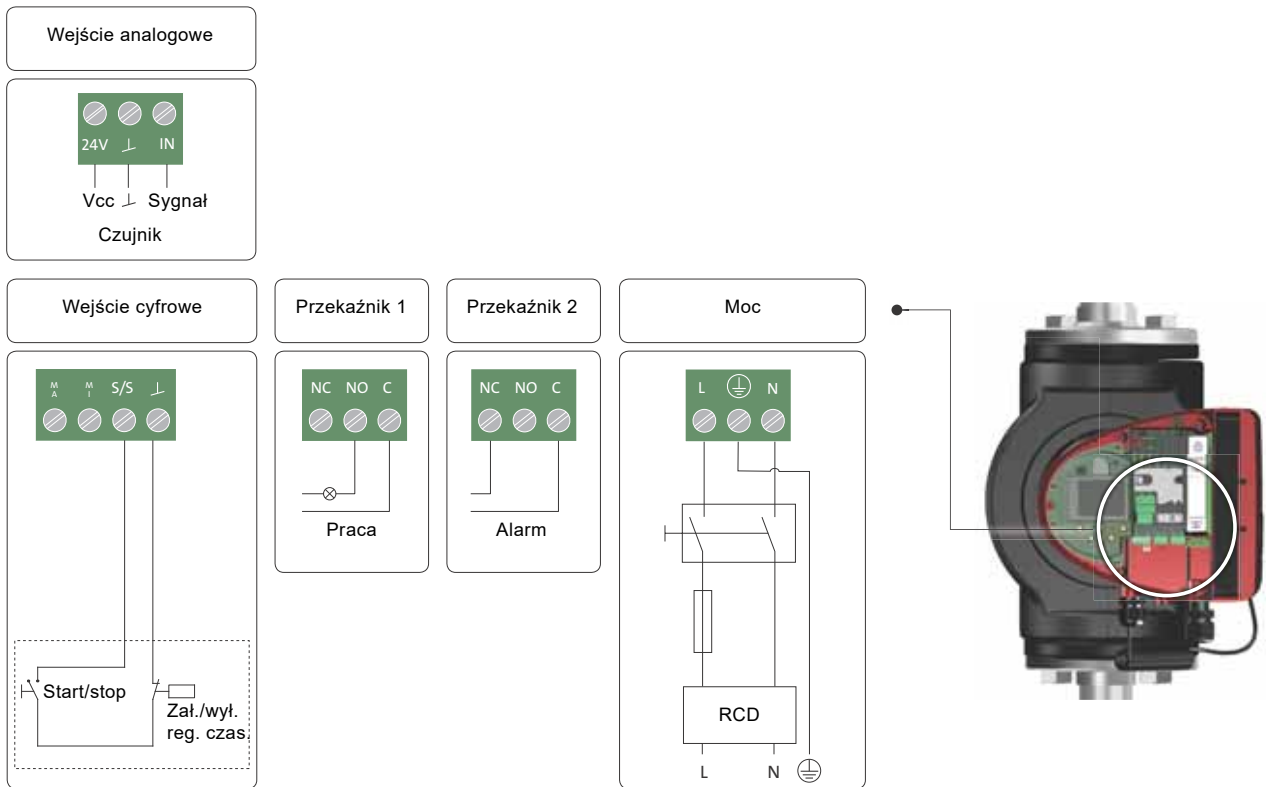
Rys. 13 Przykład połączeń w skrzynce sterowniczej dla wersji z zaciskami
