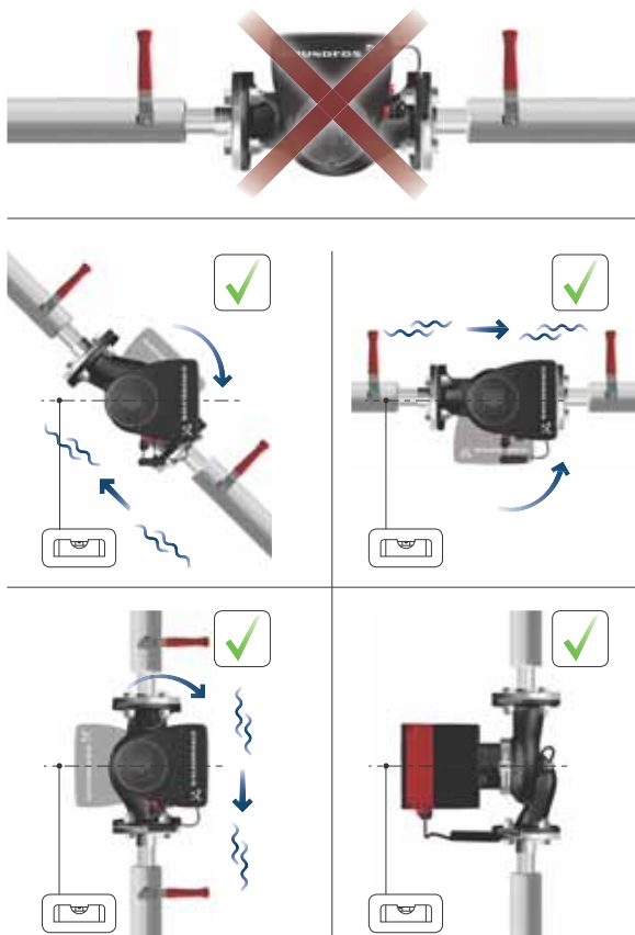
Rys. 6 Pompa ze skrzynką sterowniczą w położeniu poziomym
