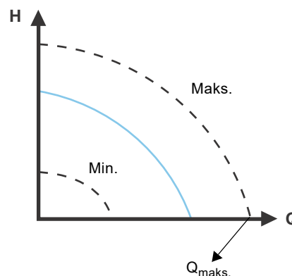
Rys. 42 Q_{\max} .
