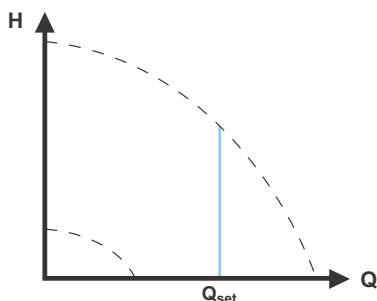
Rys. 35 Stała wydajność
